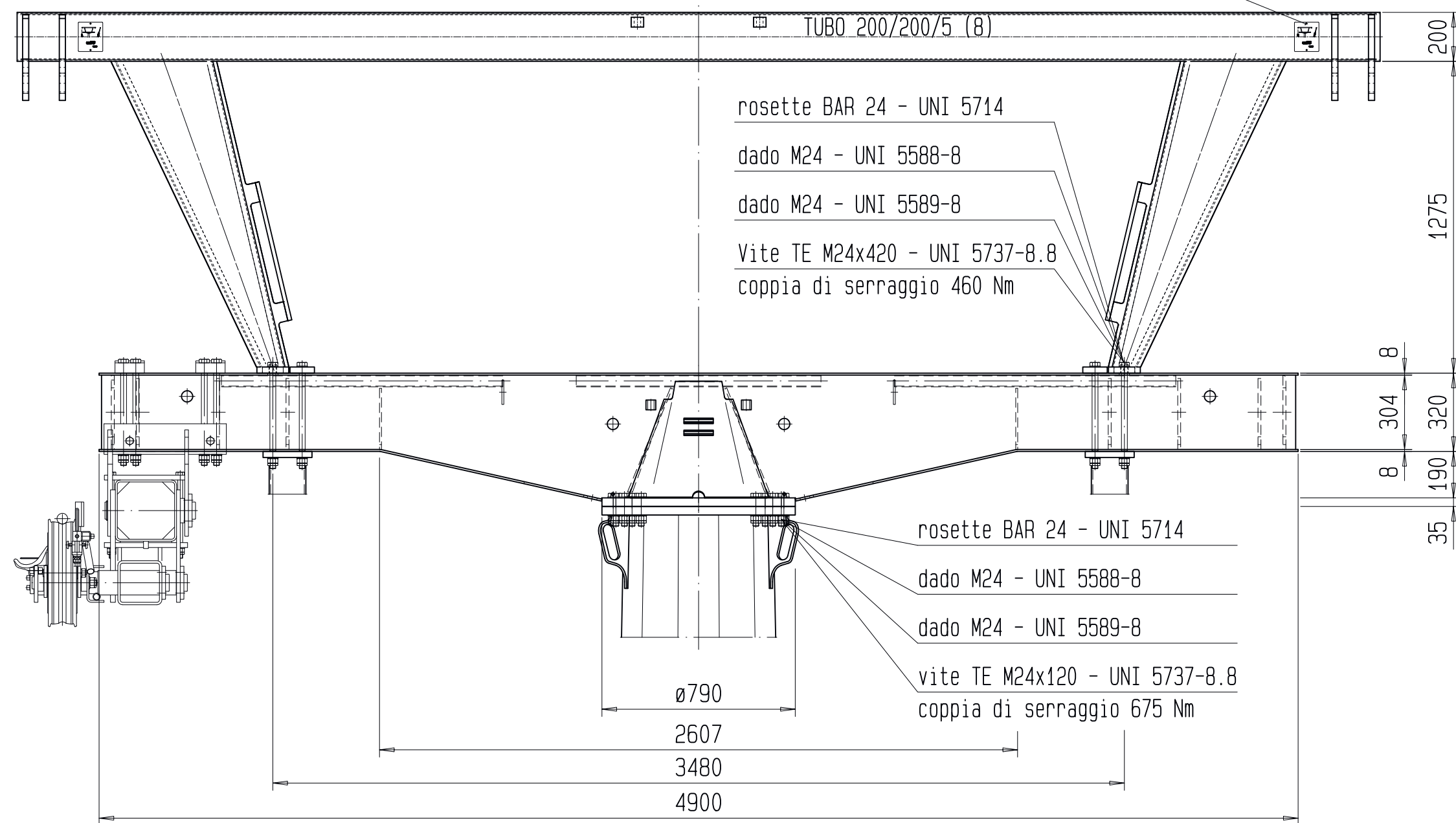
MASSAB/SCALA 1:10 ø1020 ø940 36 36 N°96 rosette BAR 24 - UNI 5714 N°48 dado M24 - UNI 5588-8 N°48 dado M24 - UNI 5589-8 N°48 vite TE M24x120 - UNI 5737-8.8 coppia di serraggio 675 Nm a = s/2 a = s a = s/2 a = s
