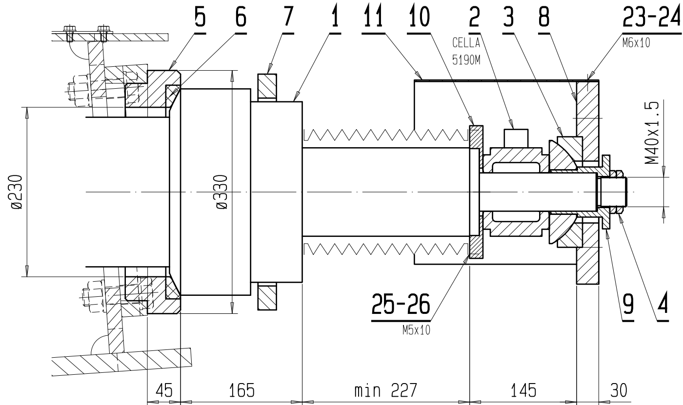
SCHNITT/SEZIONE D-D MABTAB/SCALA 1:5
