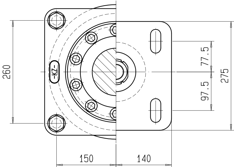
SCHNITT/SEZIONE D-D MABTAB/SCALA 1:5
