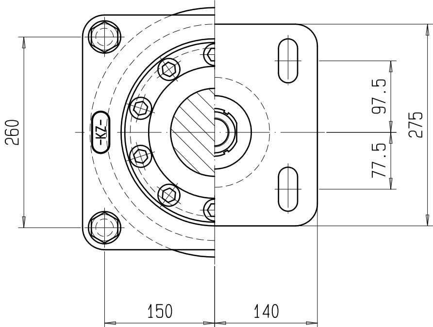
SCHNITT/SEZIONE C-C MABTAB/SCALA 1:5
