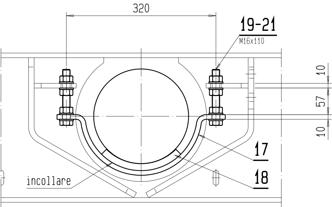
SCHNITT/SEZIONE B-B MABTAB/SCALA 1:5
