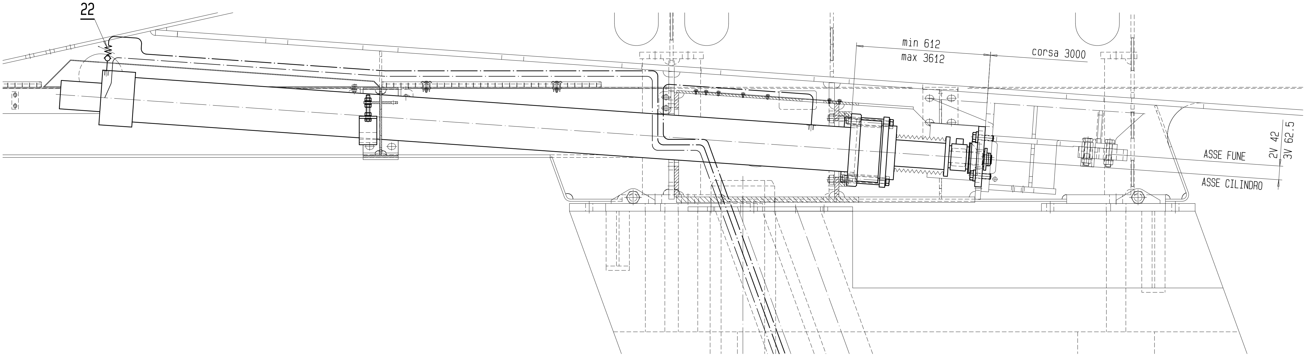
SCHNITT/SEZIONE A-A MABTAB/SCALA 1:10
