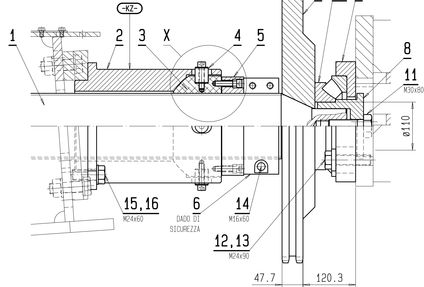
ANSICHT/VISTA D MABTAB/SCALA 1:5
