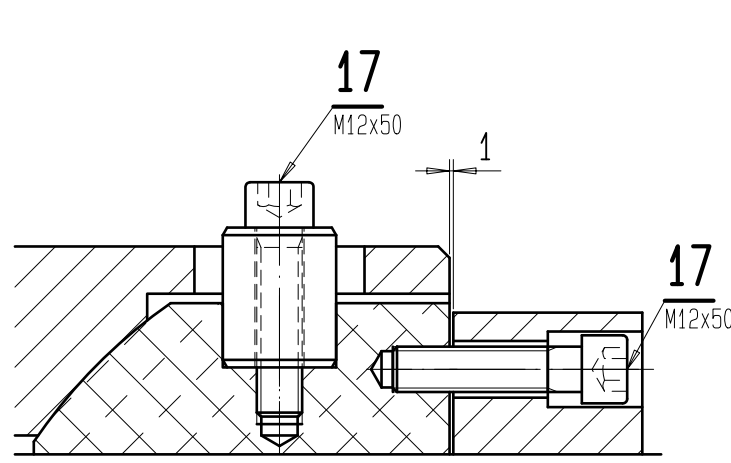
DETAIL/PARTICOLARE X MABTAB/SCALA 1:2
