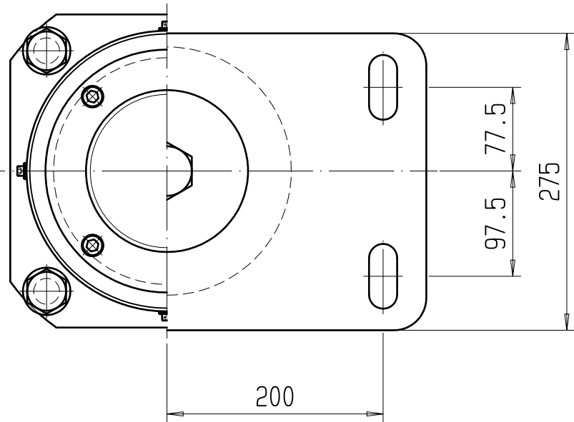
DETAIL/PARTICOLARE X MABTAB/SCALA 1:2
