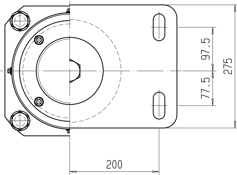
ANSICHT/VISTA D MABTAB/SCALA 1:5
