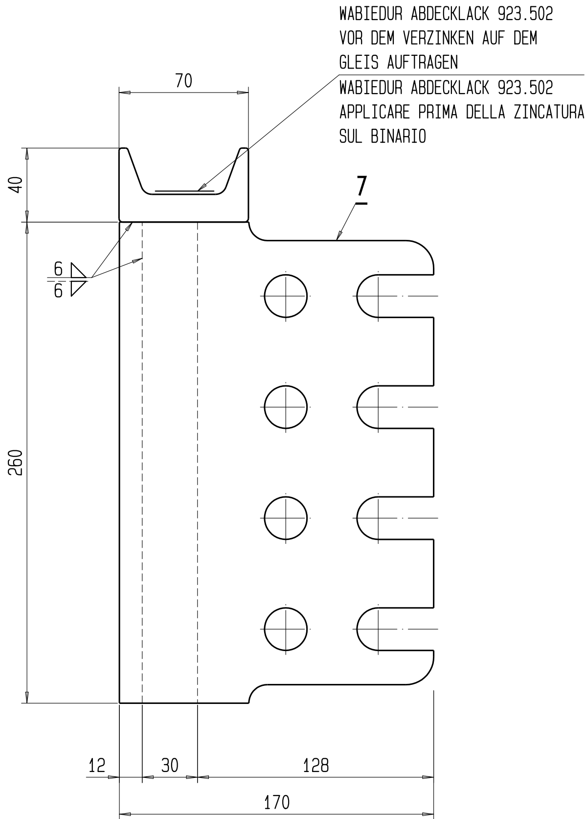
ANSICHT/VISTA A MAßSTAB/SCALA 1:2
