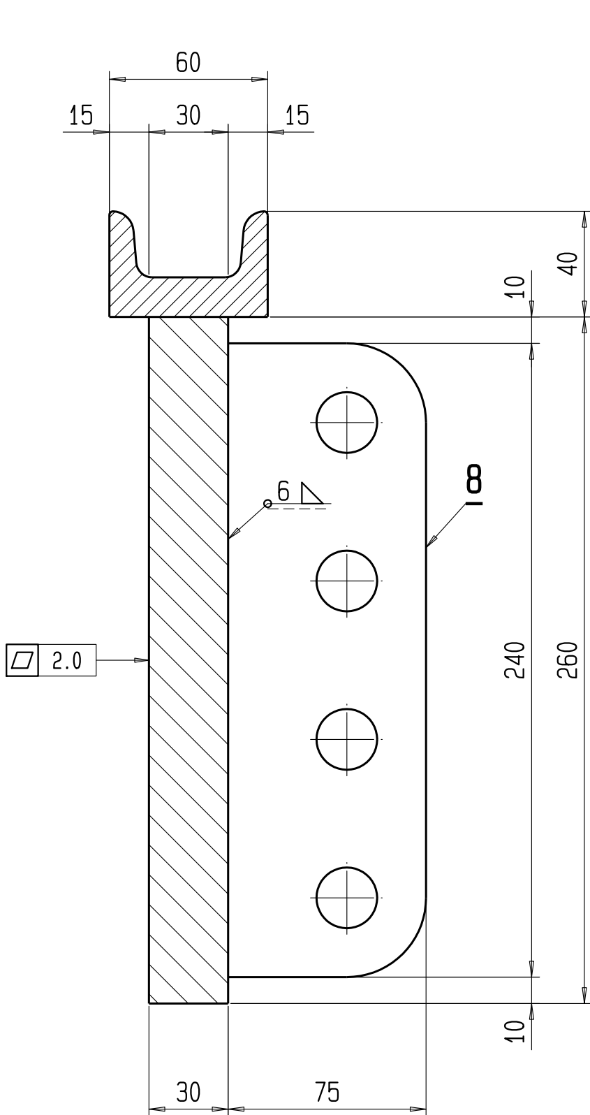
SCHNITT/SEZIONE B-B MAßSTAB/SCALA 1:2
