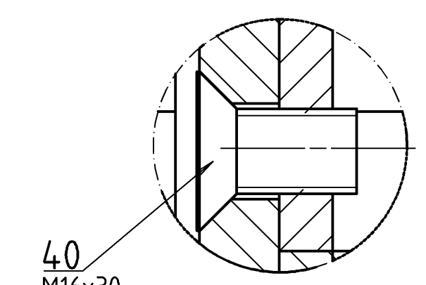
Particolare F Scala 1:1
