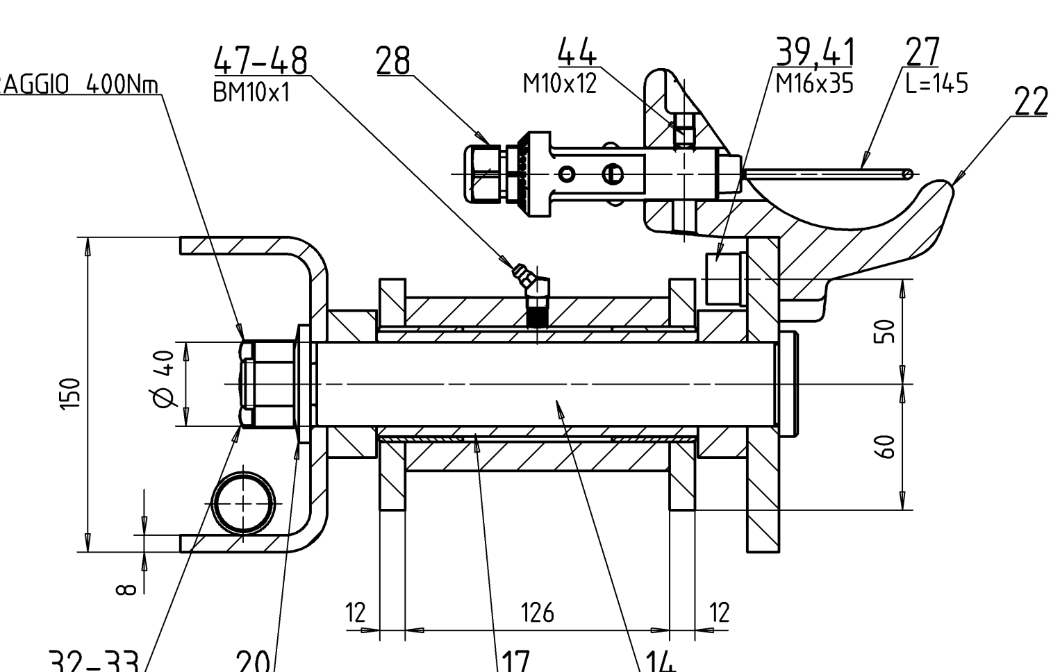
Sezione D-D Scala 2:5
