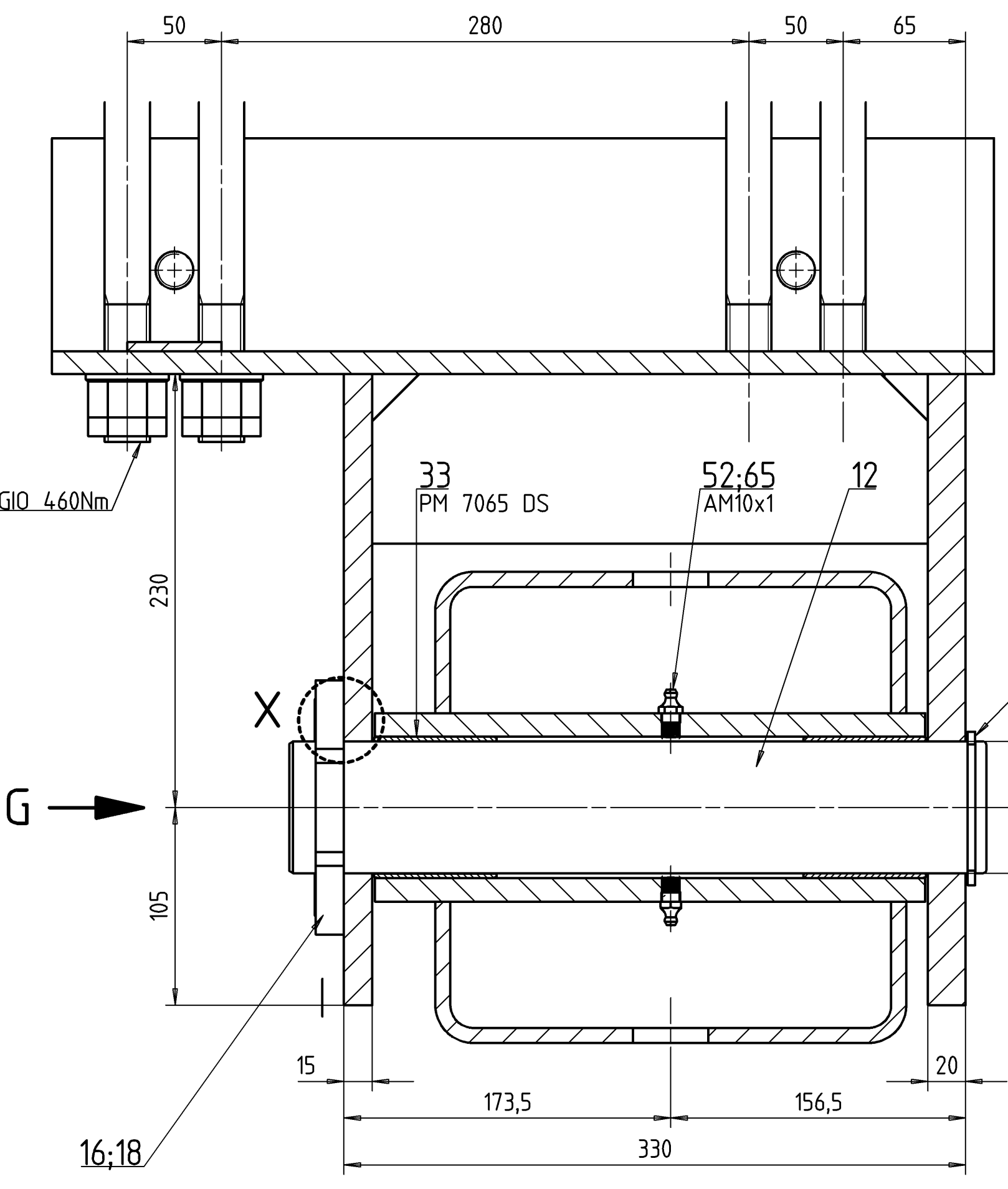
Sezione A-A Scala 2:5
