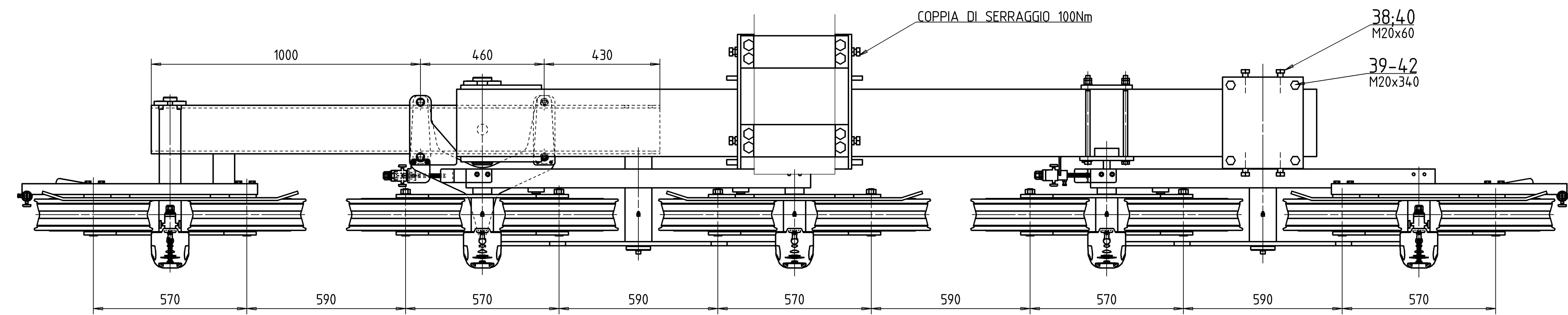
Sezione A-A Scala 2:5
