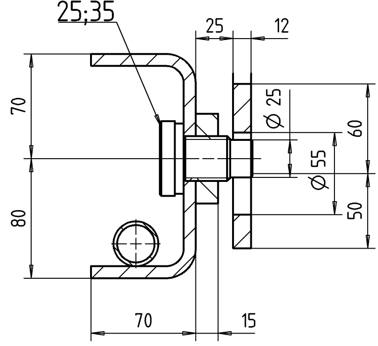
Sezione F-F Scala 2:5
