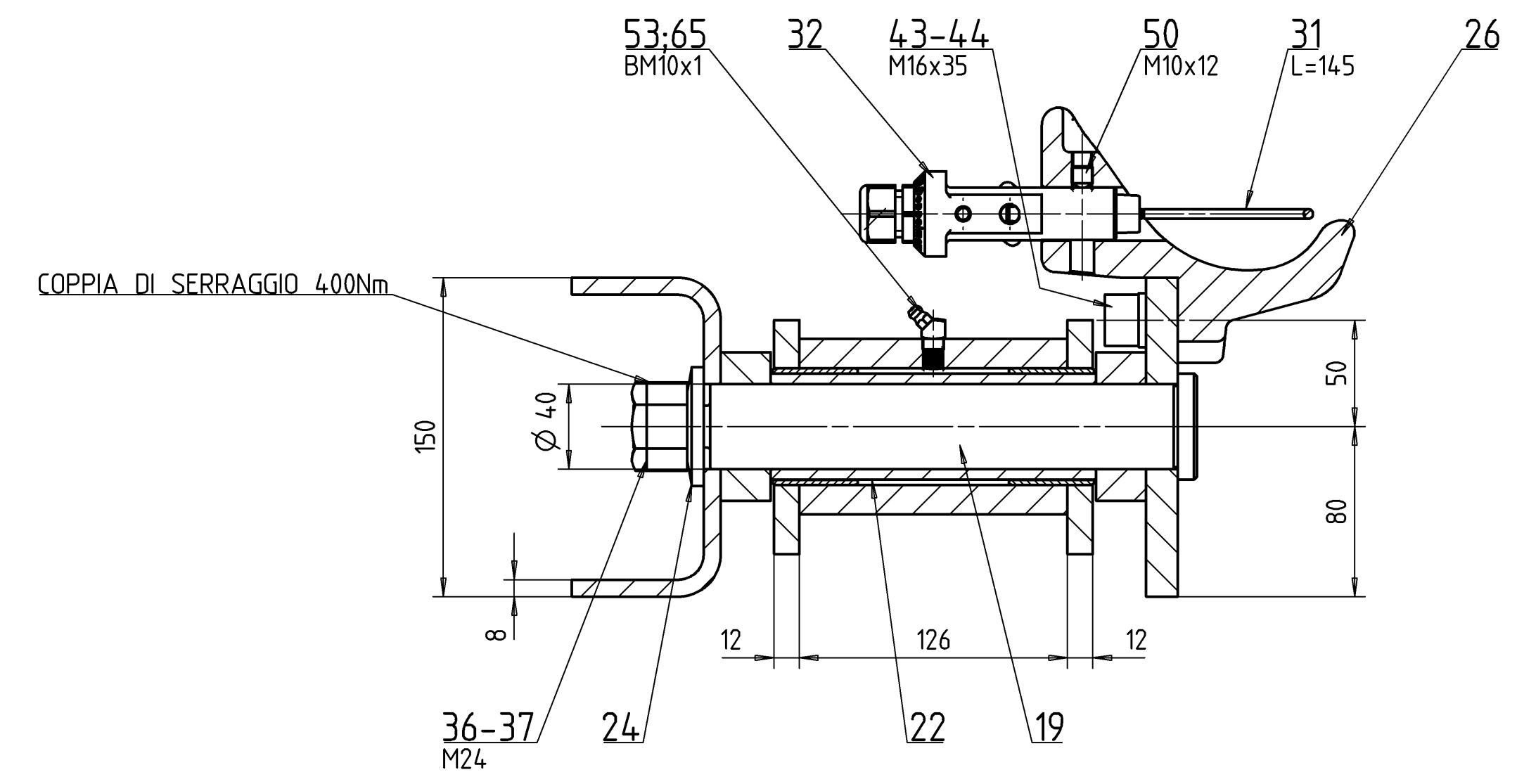
Sezione E-E Scala 2:5
