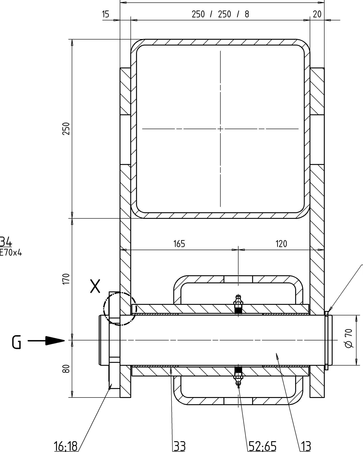
Sezione B-B Scala 2:5
