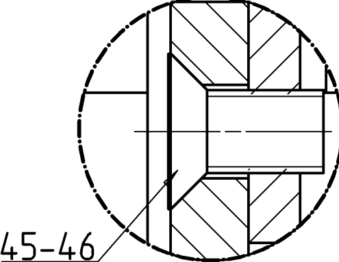
Particolare Y Scala 1:1
