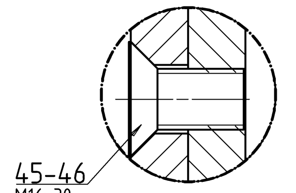
Particolare X Scala 1:1
