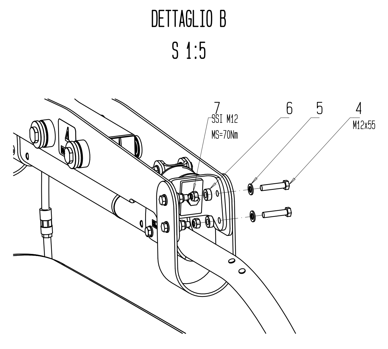
PROIEZIONE ISOMETRICA
